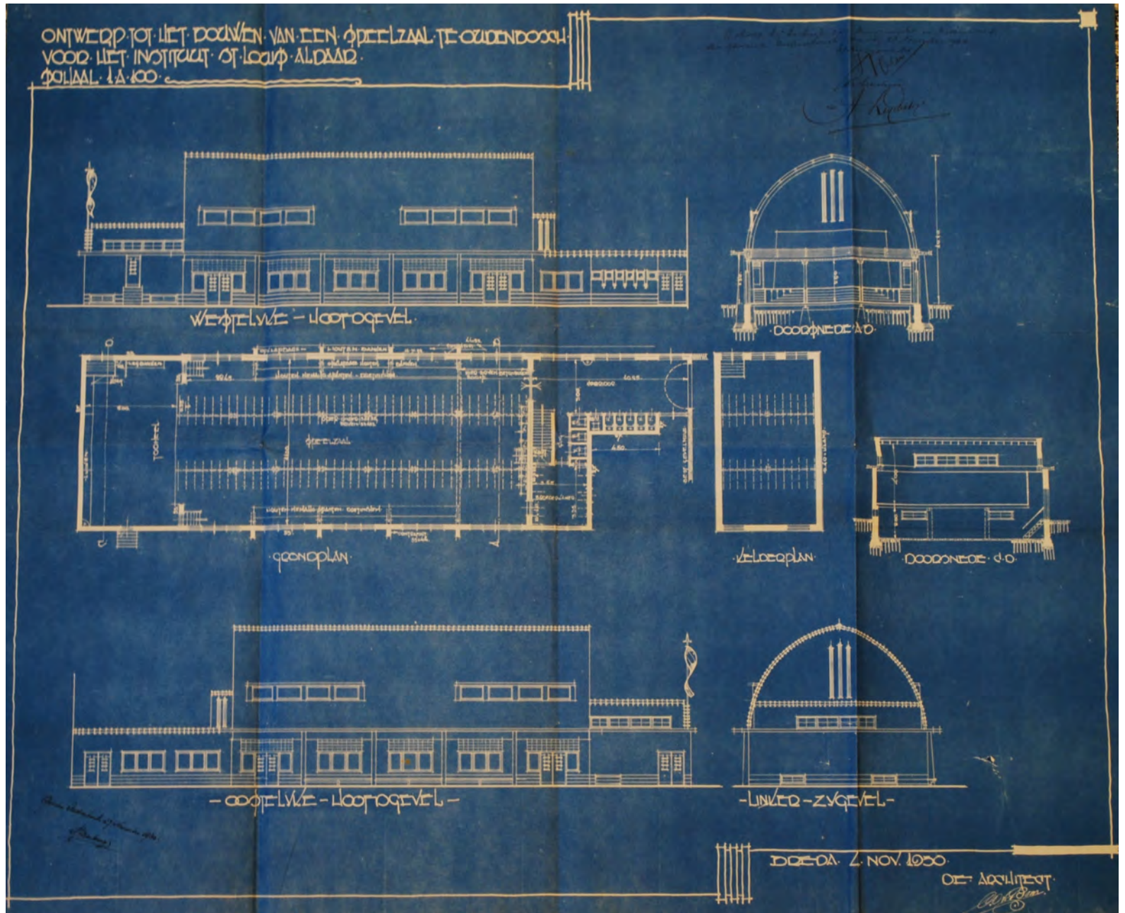
Blauwdruk van de aula (Breda 4 november 1930, ondertekend door C.A. Bom, documentatie Bernardus Wonen)
