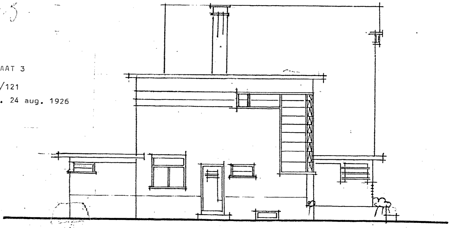
ZUGEVEL NOORD
