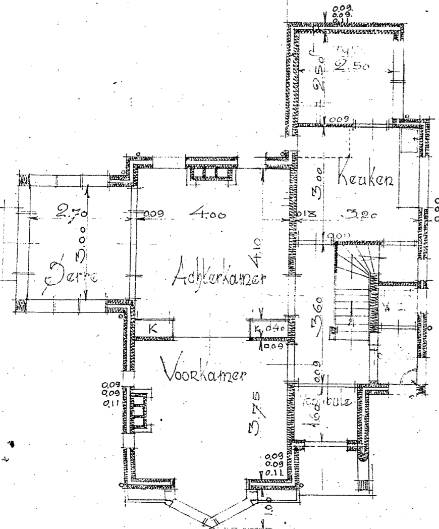
BEG. GROND
