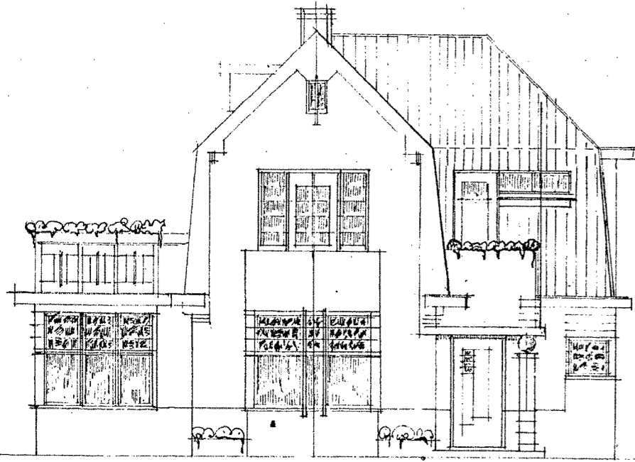
VOORGEVEL
