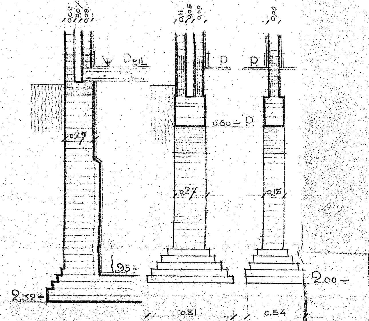
FUNDEERINGSTYPEN SCHAAL 1/20
