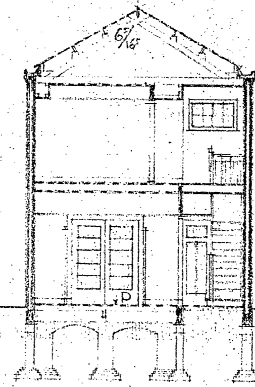
DOORSNEDEN A
