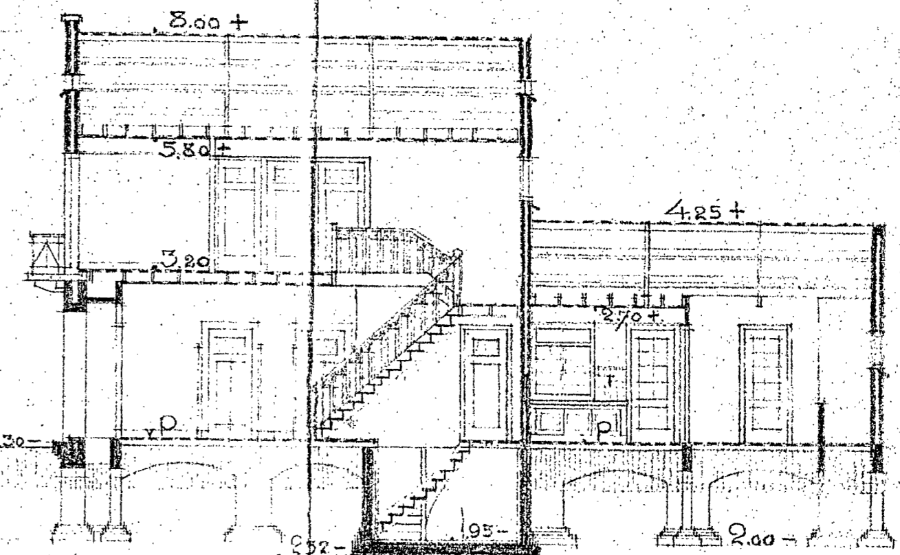
DOORSNEDEN B
