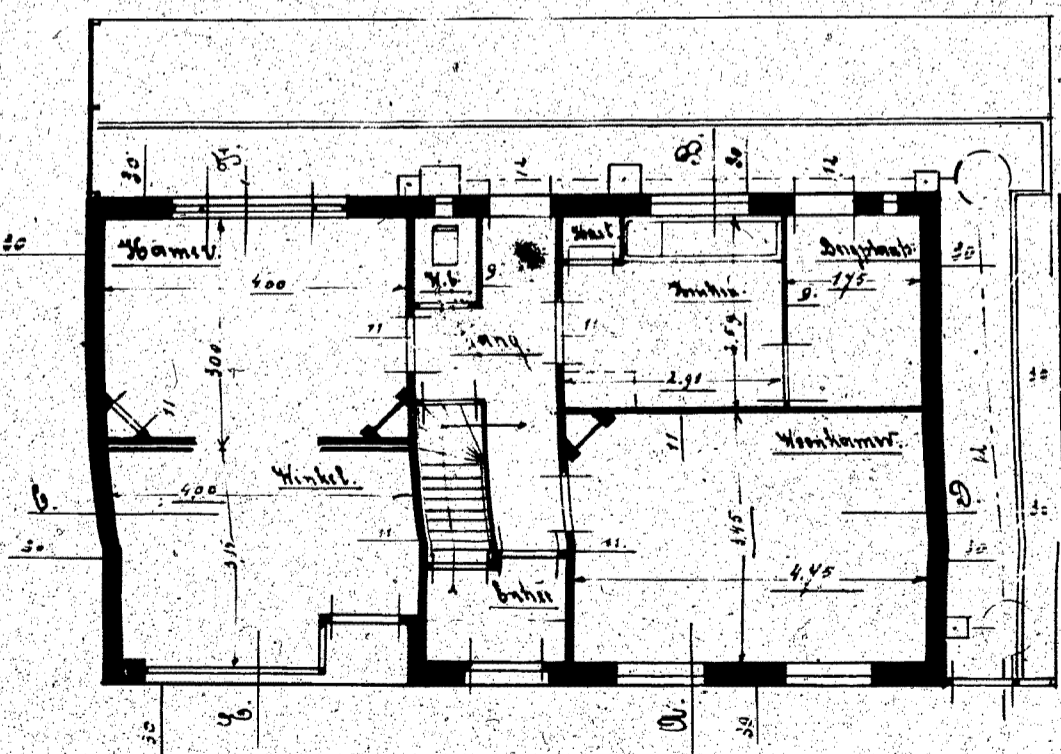
Plan Oplegbovens
