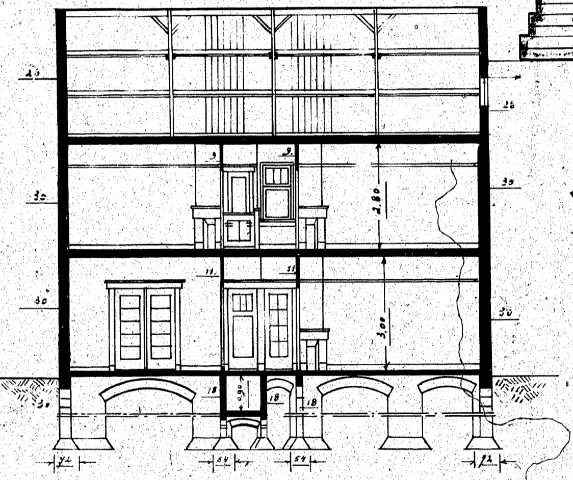
Doorsnede G.D.
