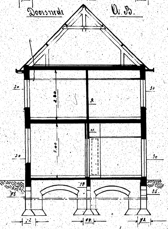
Doorsnede G.F.
