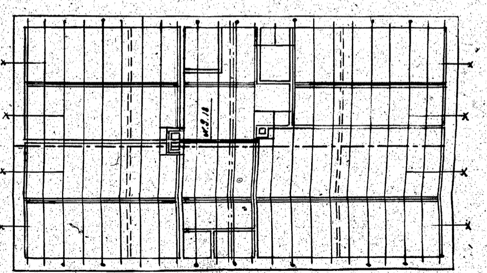
Balken bove Vindering
