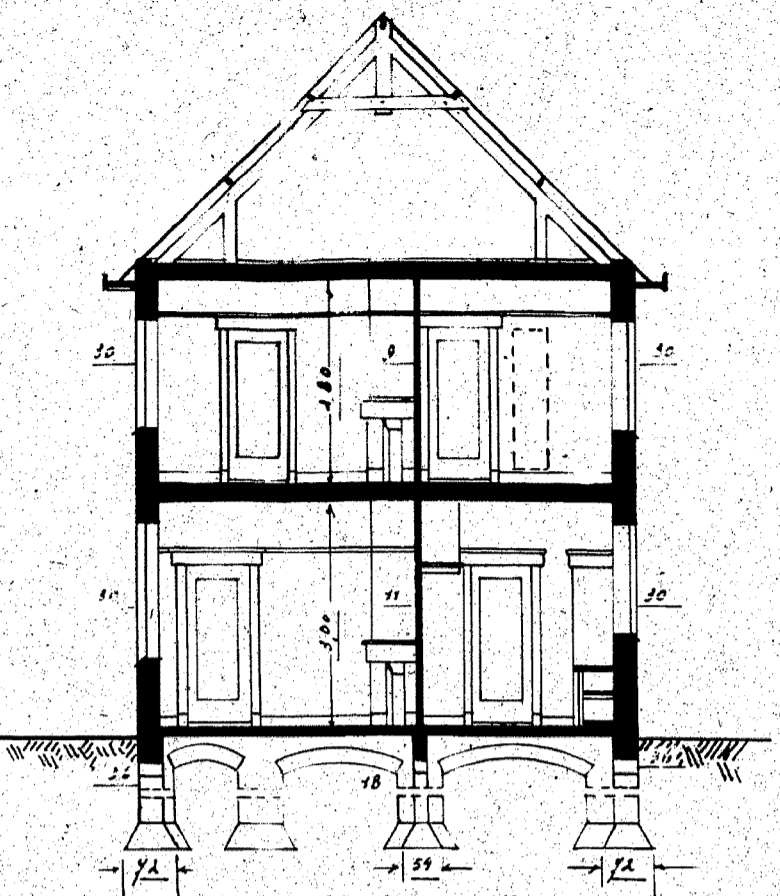
Doorsnede D. B.
