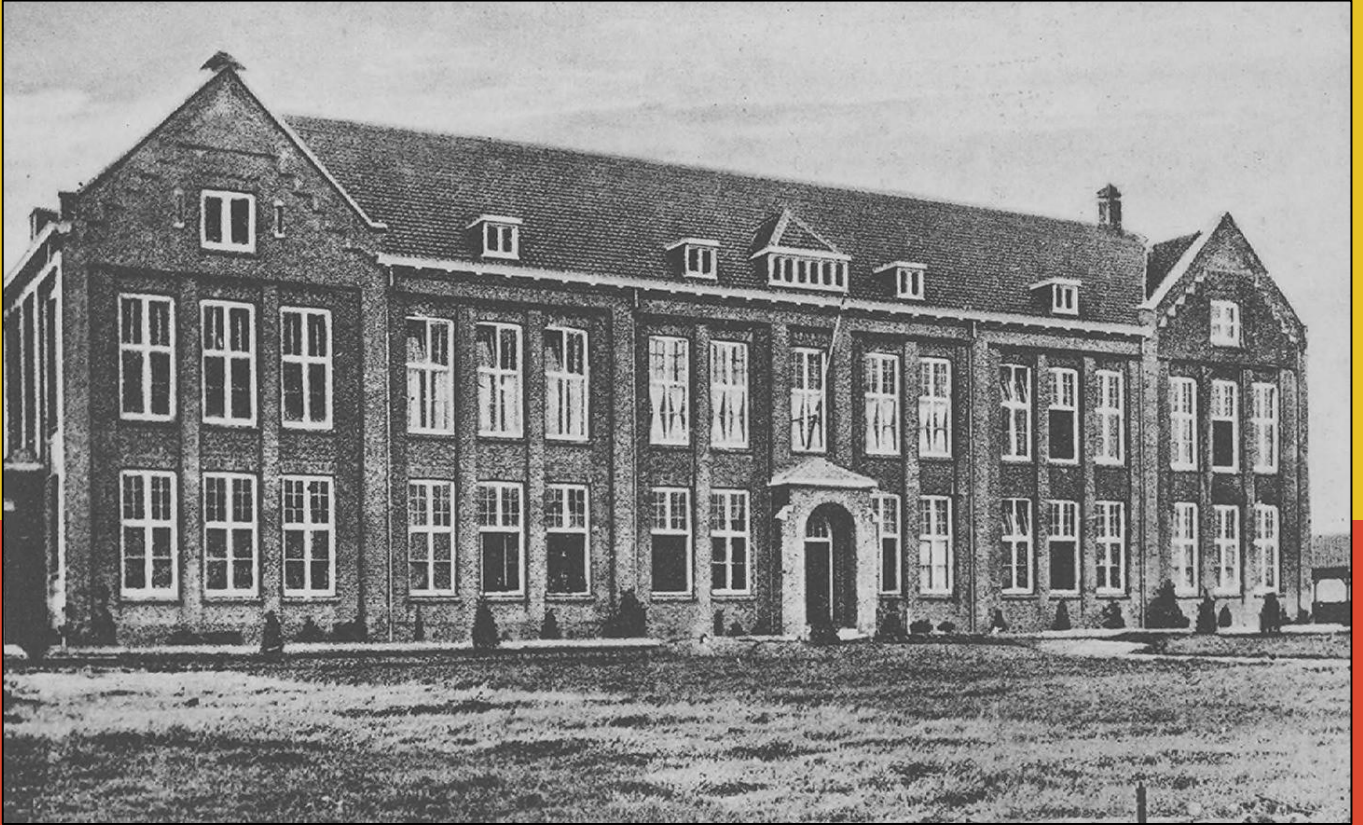
Wouwseweg (1921)
