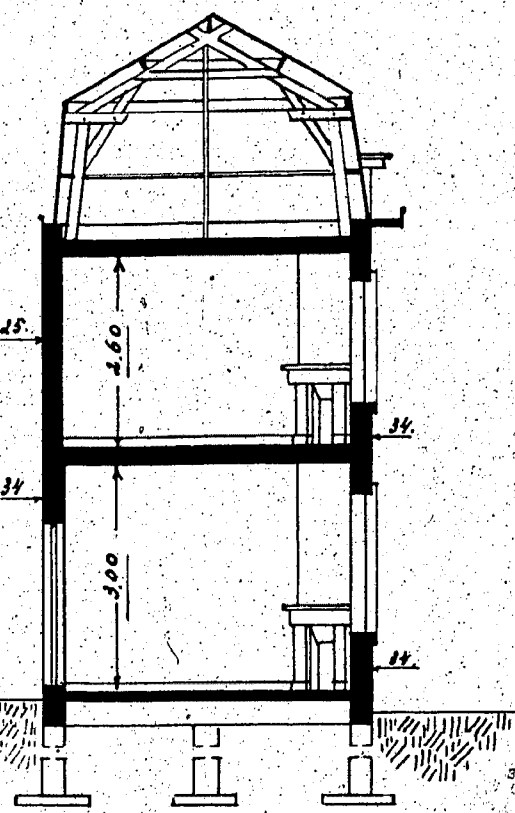
Doorsnede: A. B.
