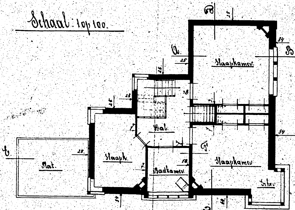
Plan van de verdieping
