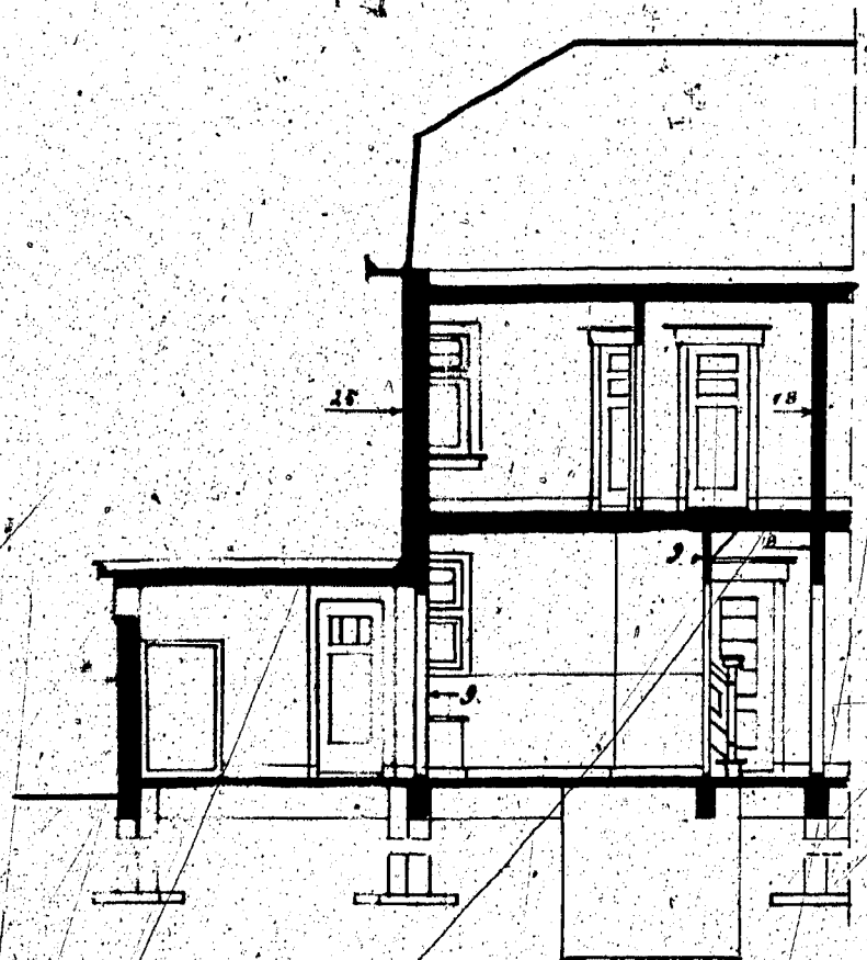
Doorsnede: C. F.
