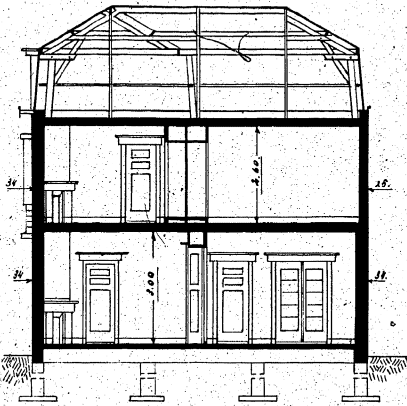
Doorsnede: C. D.
