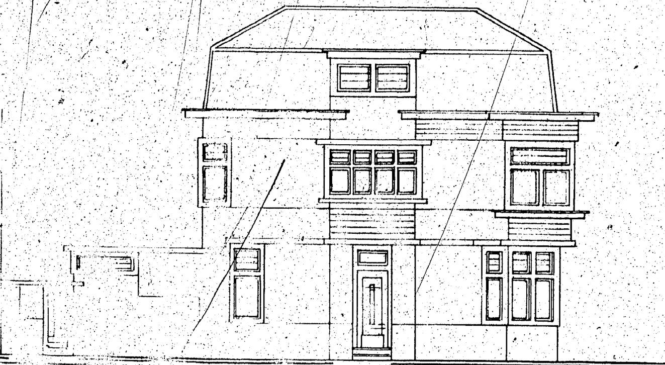
Gevel 't d. Burgem Schoonheidsstraat
