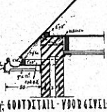
GOOTDETAIL - VOORGEVEL.
