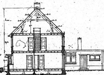
STORFBEDE A...
