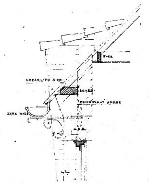
GEWAZIGDE GOOTDETAIL
