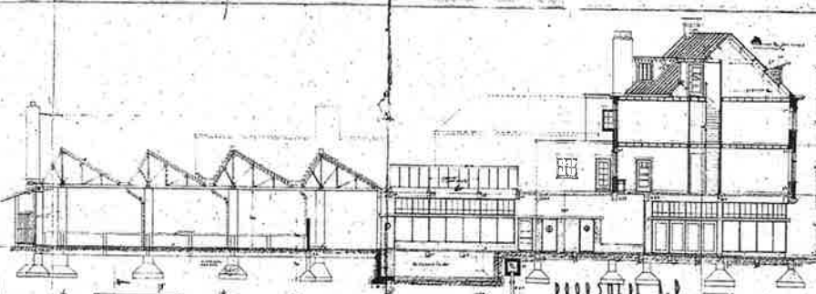
DOORSNEDEN A.D.
