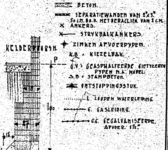
ZIJGEVELS TOELICHTING
