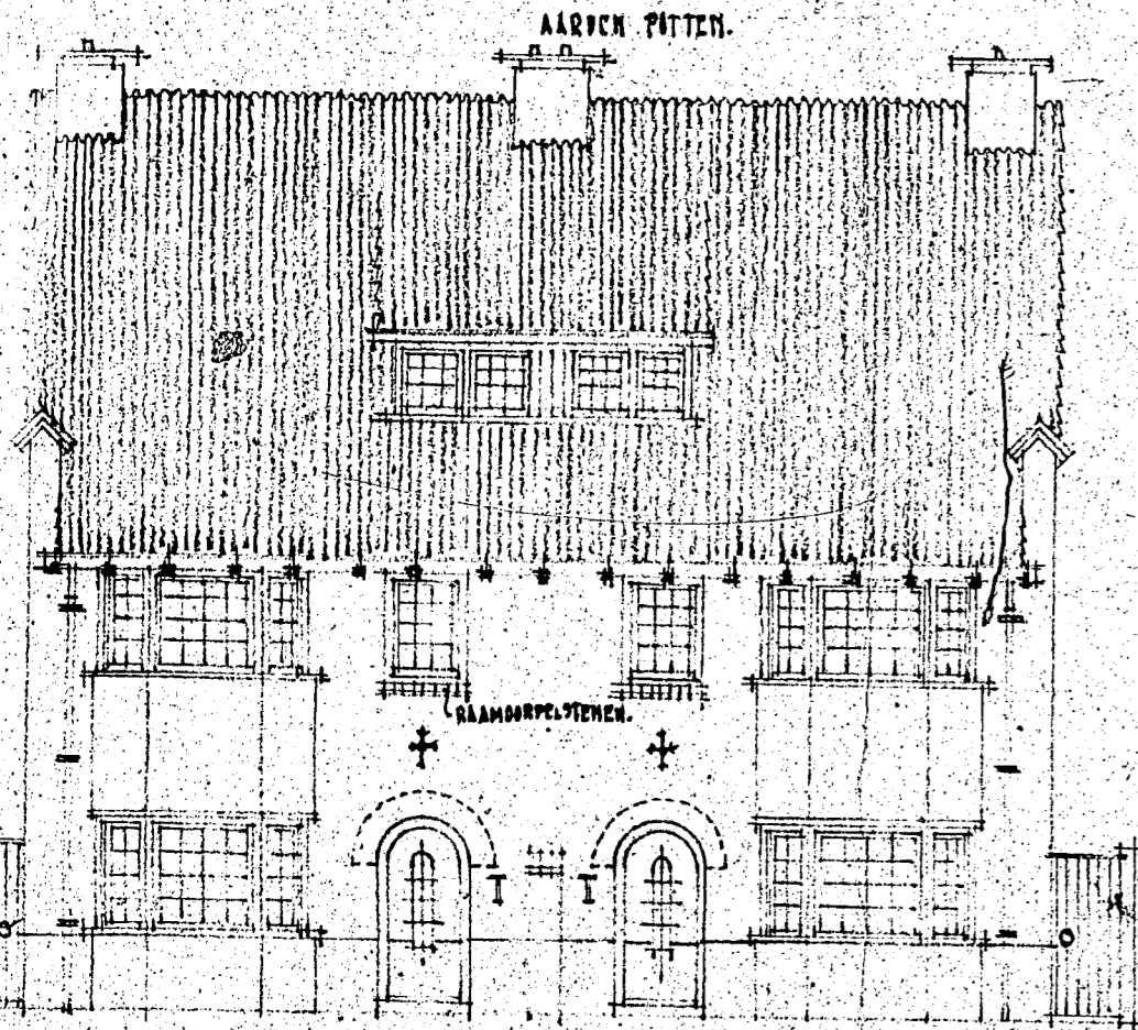
VOORGEVEL
