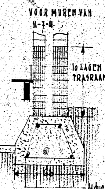
TUNDERINGSTYPEN 1:10
