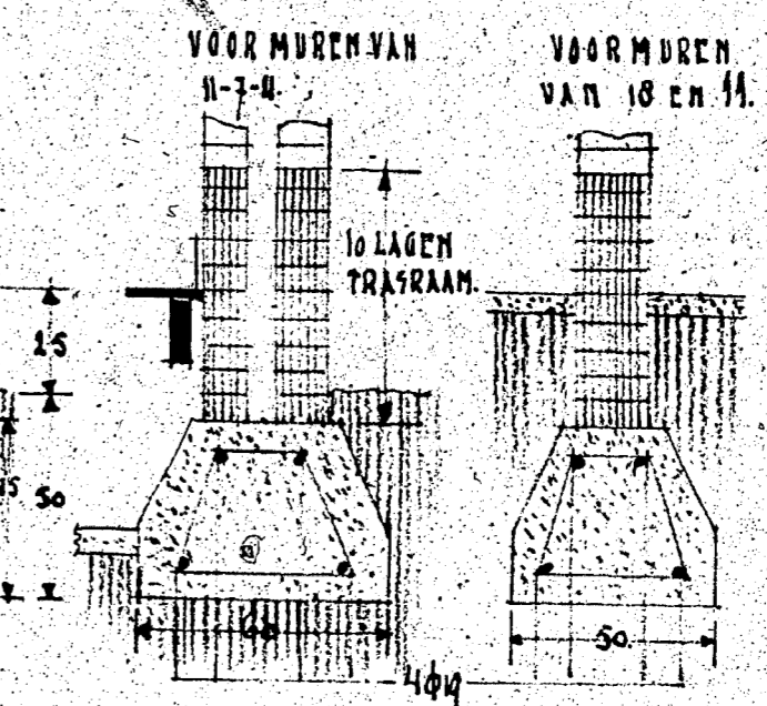
TUNDERINGSTYPEN 1:10
