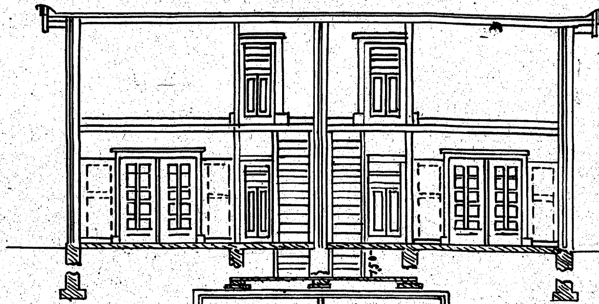
Schaal 1:100
