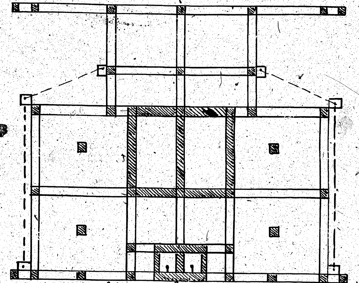
Schema der Fundering
