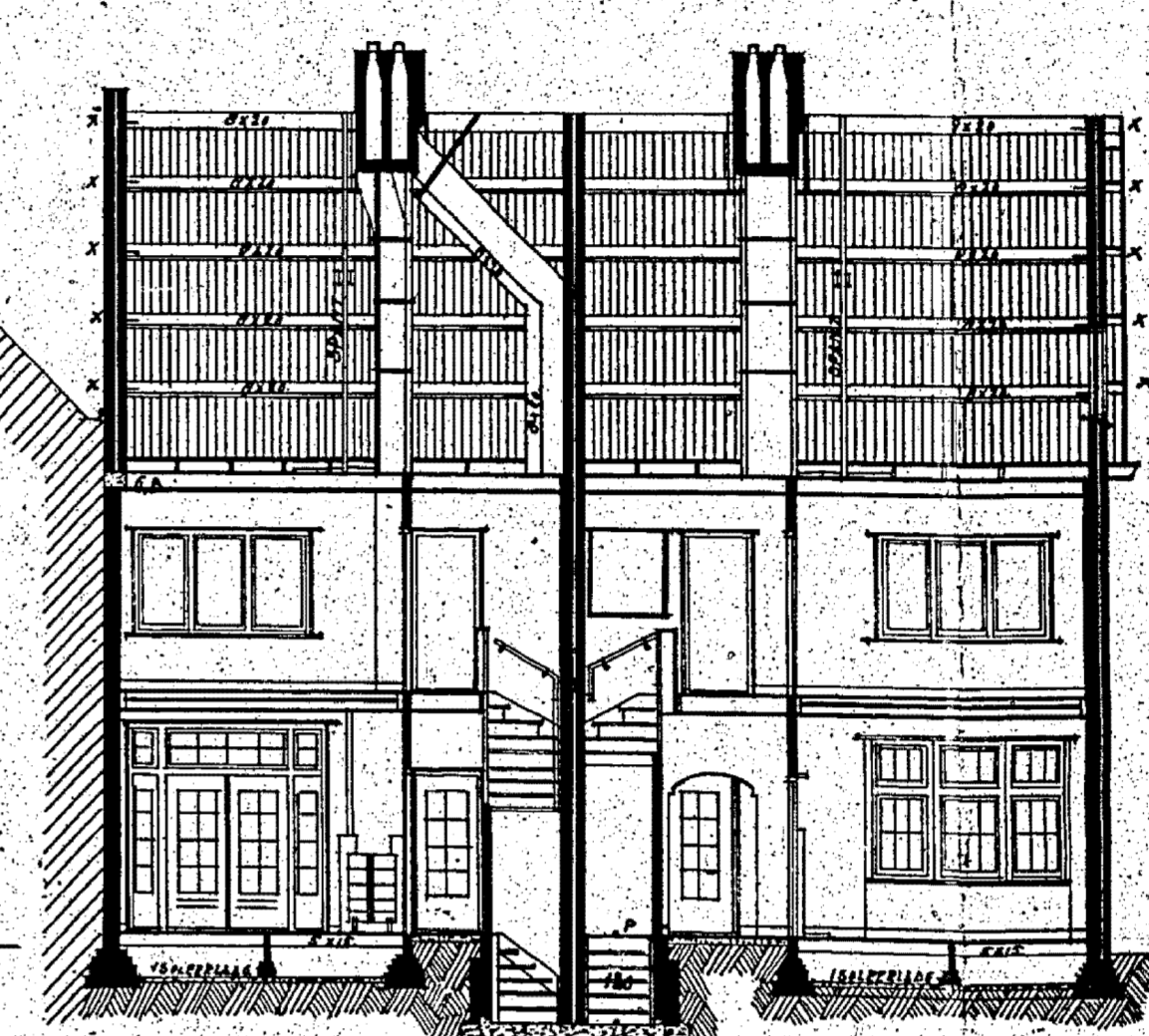
DOORSN. B-B
