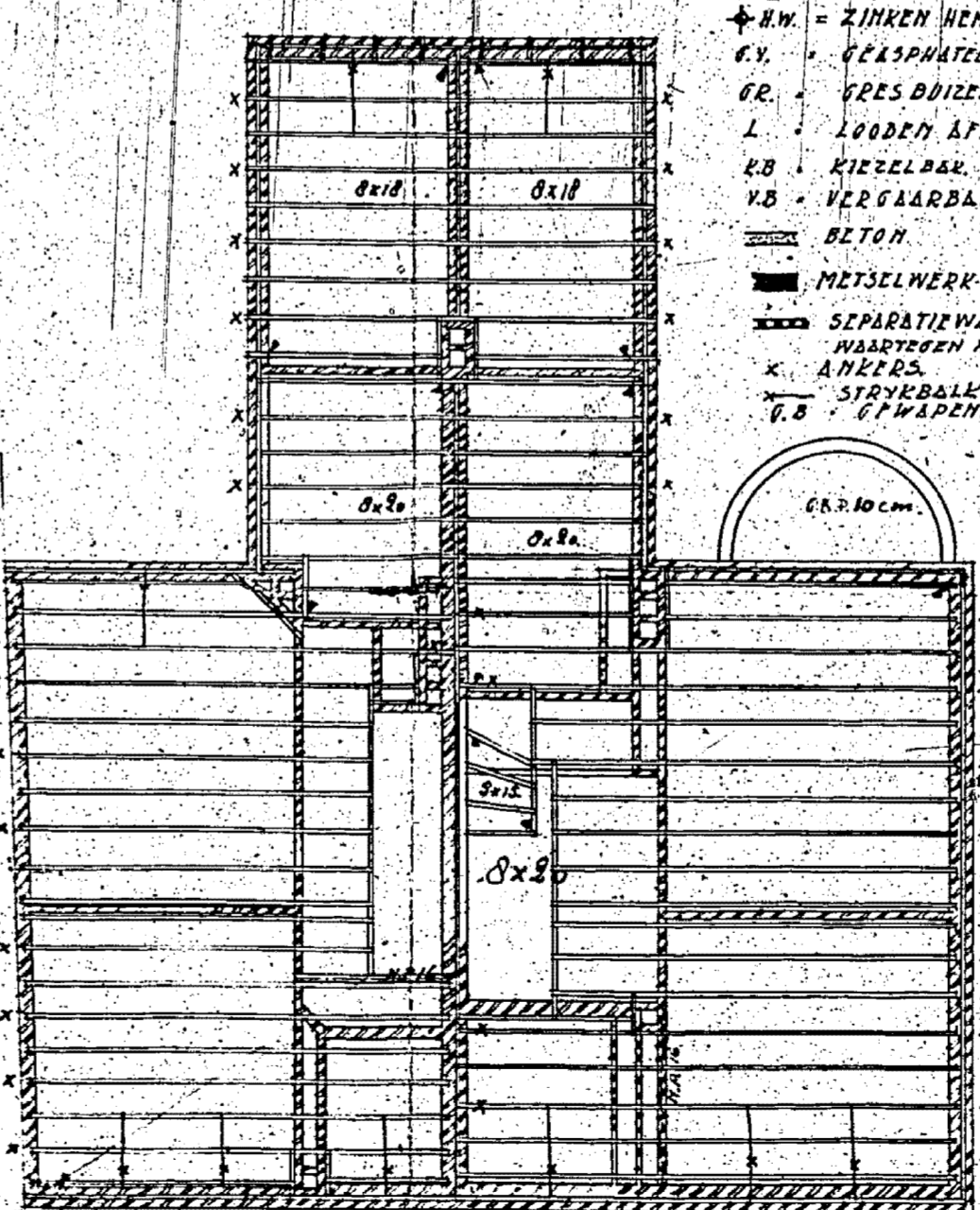
TWEEDE BALKLAAG
